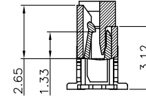
SECTION A-A SCALE 1:1
