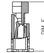
SECTION A-A SCALE 1:1
